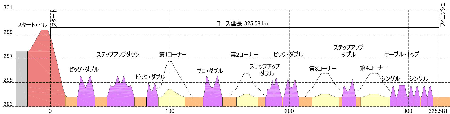
BMXコース縦断図
